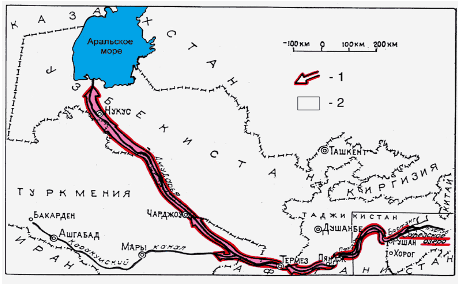
Рис.1. Обзорная схема возможной зоны поражения селевыми потоками в случае прорыва Сарезского озера.
