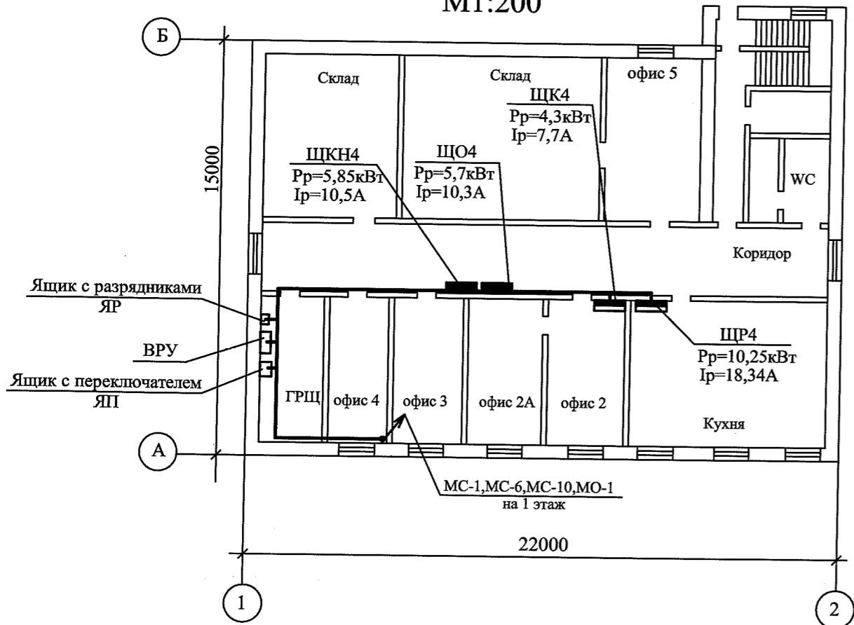
План подвала M1:200
